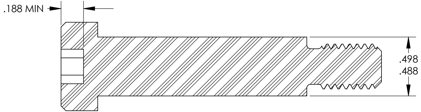
SECTION A-A
